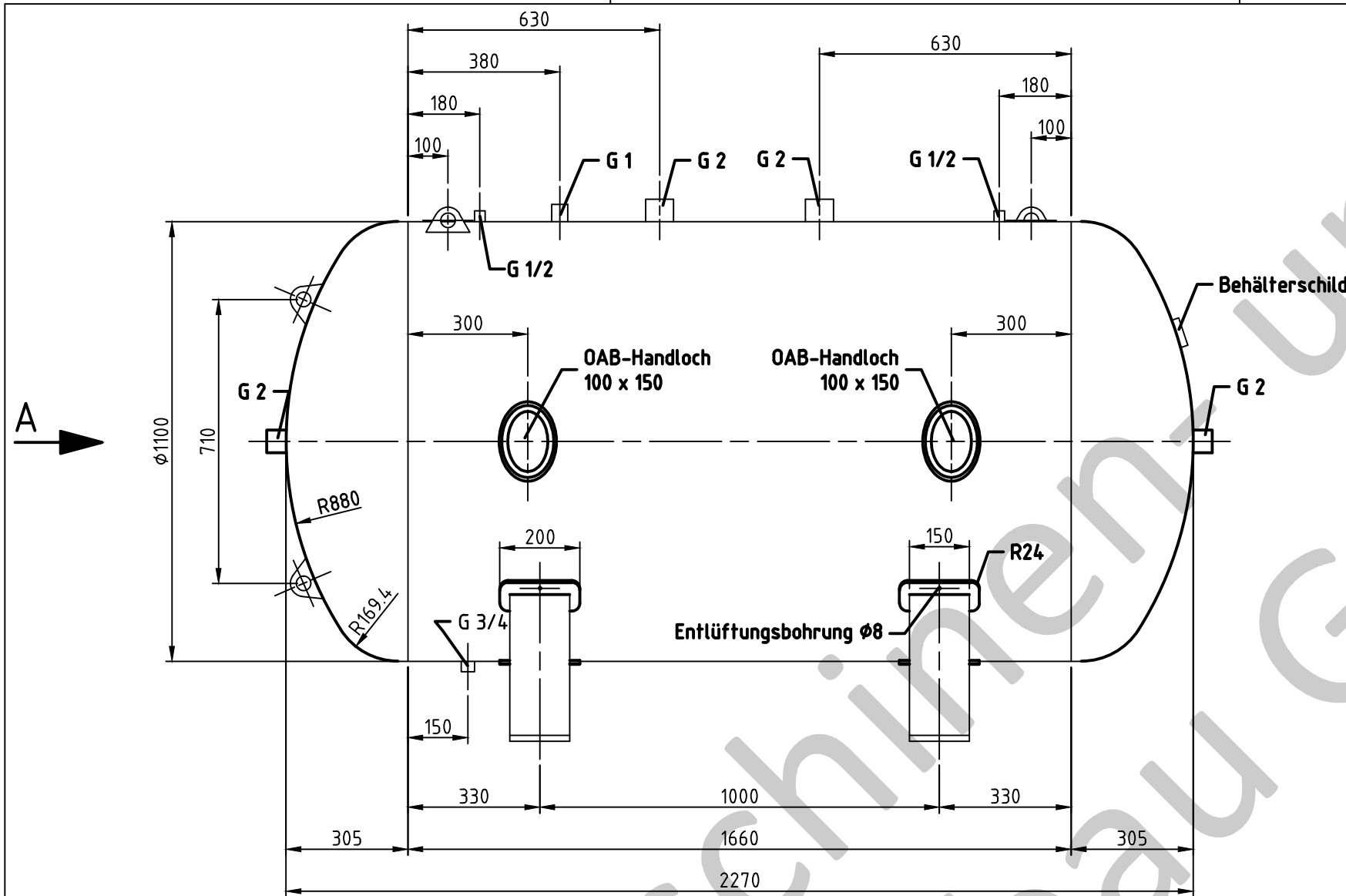
Ansicht A
